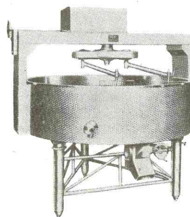
Vasca polivalente in acc. inox da lt. 2000 a lt. 7500 per formaggi
