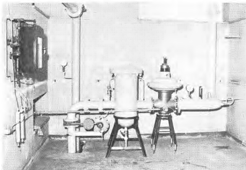
Interno della cabina di via Trigolo. Veduta generale delle apparecchiature, per riduzione di 1° salto da 40 Ate a 3,5 Ate sono ben visibili i filtri scambiatori di calore; i riduttori con monitor pilotati automatici; valvola di sfioro a contrappeso).
