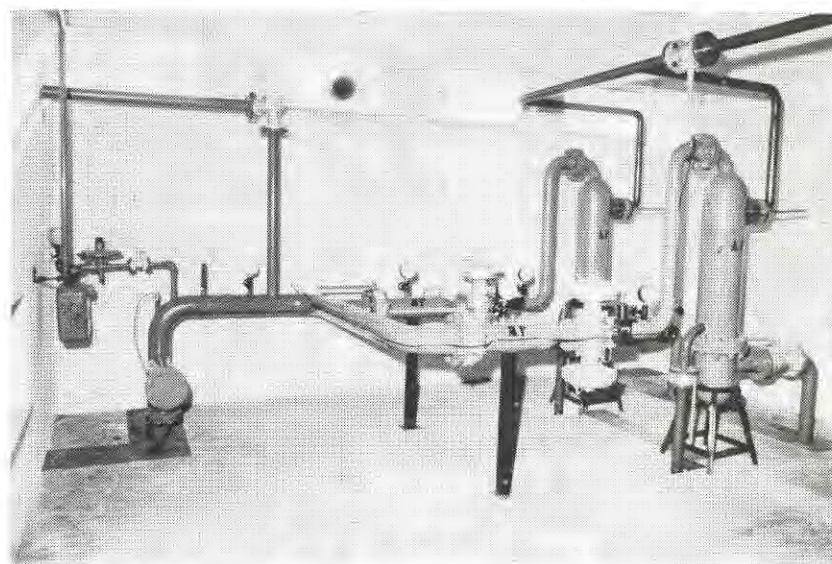
Interno della cabina di via Stadio. Veduta parziale delle apparecchiature di riduzione di 2° salto (valvola di blocco a comando pressostatico; filtro depuratore atto a trattenere pulviscolo sino a 5 micron; indicatore di intasamento; riduttore per misura venturimetrica; registratore triplo di portata, temperatura e pressione).
