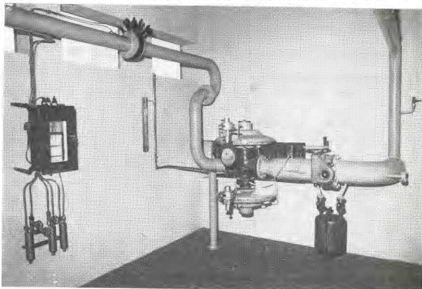
Interno della cabina di via Piave. Veduta parziale delle apparecchiature di riduzione di 2° salto (riduttore con monitor, piloti automatici ad incremento orario della pressione; registratore triplo di portata, temperatura e pressione; odorizzatore a lambimento; saracinesca di uscita).
