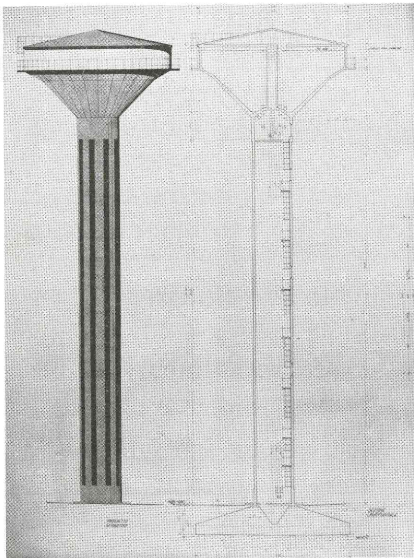
Il progetto della nuova torre-acquedotto.
