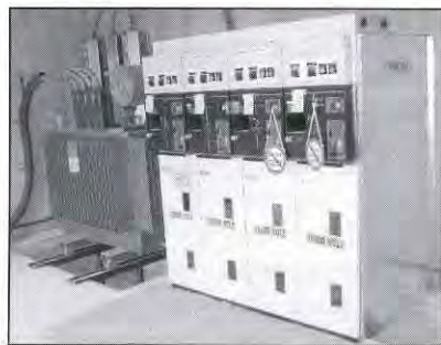
Nuova cabina elettrica nel 3° lotto del Piano Insediamento Produttivo.
